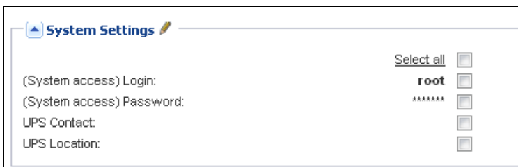
Abbildung 75. Knotenkonfigurationsbereich
