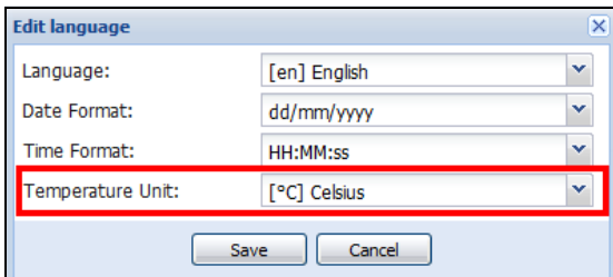
Abbildung 14. Spracheinstellungen bearbeiten
